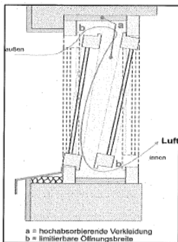
Konstruktionsprinzip „HafenCity-Fenster“
