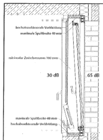
Umsetzungsbeispiel „HafenCity-Fenster“
